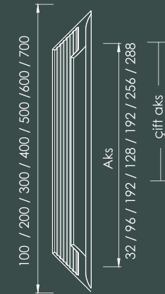
■ Alm. (L) LINE MINI GAMA EKS.8080
