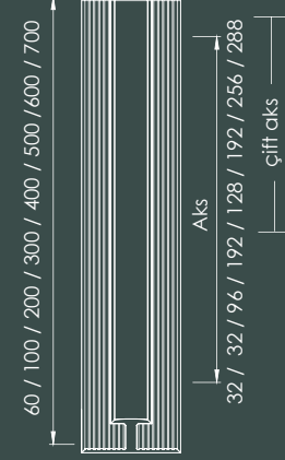
■ Alm. (H) LINE MINI BETA Duo EKS.8073
