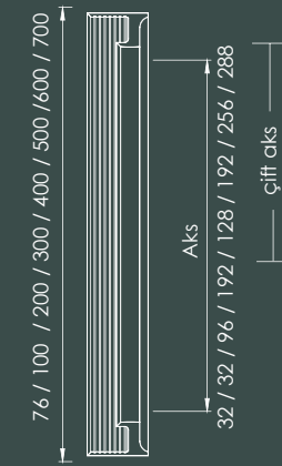
■ Alm. (L) LINE MINI BETA EKS.8078
